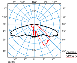
Publisca P1W-AB2L-LRA/1200-730 2G1S ET (CLO initial value)
