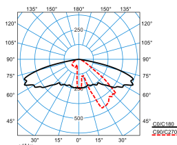
Publisca P1W-AB2L-LRA/1200-730 2G1S ET (CLO end value)
