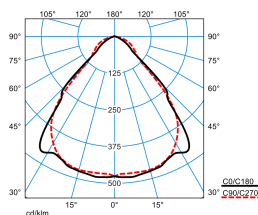
SFlow C3-L MRW LED4000-8TW ETDD8 LLWS 01 (DSU)
