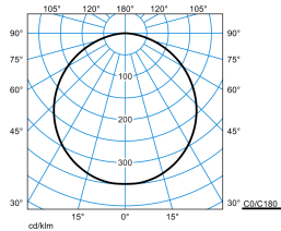
Olisq RWD4 DW 40-830 ETBLE +CAS-S IP54 + Olisq RWD4 ZDR 1/1 05
