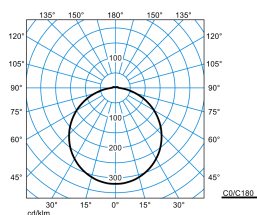
Olisq RWD4 DW 40-830 ETBLE +CAS-S IP54 + Olisq RWD4 C 01
