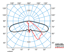
Publisca P1-AB2L/2000-740 3G1S ETDD (CLO initial value)
