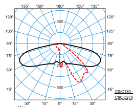
Publisca P1-AB2L/2000-740 3G1S ETDD (CLO end value)
