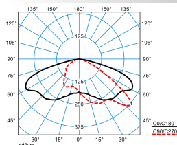
LnPlus 40-AB7L-SLR1/3200-730 4G1 ET (CLO initial value)
