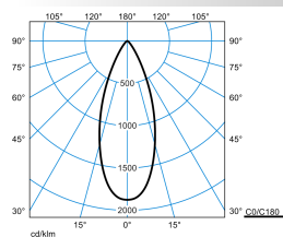
Altigo G2 60 RB17L/1800-830 1G1P + VE IP66 24V DC 250W
