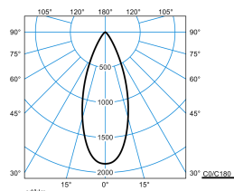
Altigo G2 60 RB17L/1800-830 1G1P + G2 VE IP66 24V DC 80W
