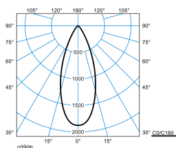
Altigo G2 60 RB17L/1800-830 1G1P + G2 VE IP66 24V DC 240W
