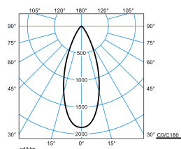
Altigo G2 60 RB17L/1800-830 1G1P + G2 VE IP66 24V DC 30W
