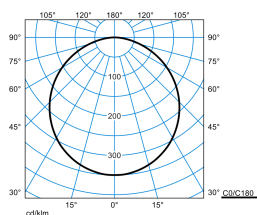
Olisq RWD2 DW 20-840 ETBLE +CAS + Olisq RWD2 ZVF 01
