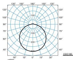
Olisq RWD2 DW 20-840 ETBLE +CAS + Olisq RWD2 ZDR 1/2 01
