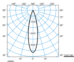
E-Line PRO 78 Lentyp L-MF 30-830 M33 ET 03 Blank
