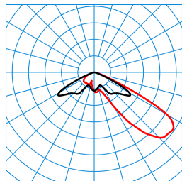
LnPlus 70-AM19L/38000-730 36G1 ETDD (CLO end value) TX390181 ■ C0 - C180 ■ C90 - C270 DIN 5040: A30 UTE: 1,00 J DLOR: 100 % ULOR: 0 % CEN Flux Code: 26 78 99 100 100
