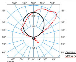
Luceos S G3 PAW-IA 170-8TW ETDS FU 01 (DWW)
