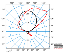
Luceos S G3 PAW-IA 170-8TW ETDS FU 01 (DSU)
