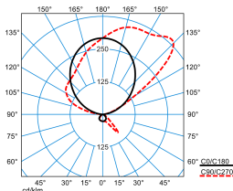
Luceos S G3 PAW-IA 170-8TW ETDS FU 01 (DCW)
