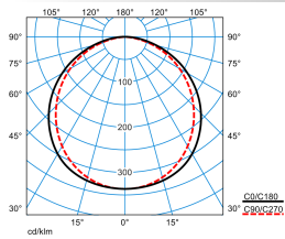
Linell 3PID10 DW-F 21-940 ETDD 01
