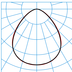
Lunexo D2 CDP-I 5500-8TW ETDD8 01 (DCW) TX872961 C0 - C180 C90 - C270
