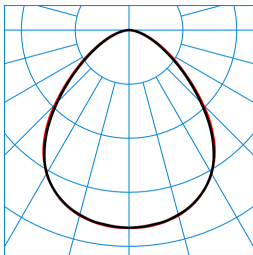
Lunexo D2 CDP-I 5500-8TW ETDD8 01 (DWW) TX872963 C0 - C180 C90 - C270
