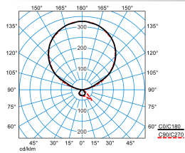
Luceos S G2 PAW-IL 150-840 ETDS 01 TX299603
