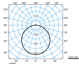
Olisq RWD4 DW 40-830 ET EB3 + Olisq RWD4 ZDR 1/2 03
