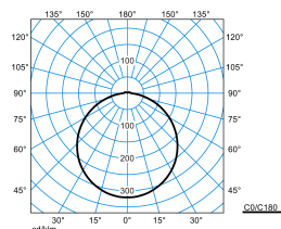
Olisq RWD4 DW 40-830 ET EB3 + Olisq RWD4 C 01
