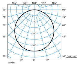
Olisq RWD3 DW 50-830 ET EB3 PC + Olisq RWD3 ZDR 1/1 03
