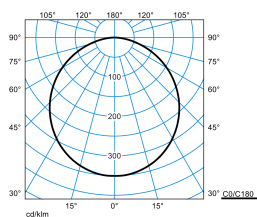
Olisq RWD3 DW 50-830 ET EB3 PC + Olisq RWD3 ZVF 05
