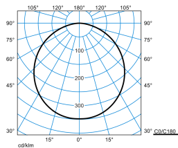
Olisq RWD3 DW 50-830 ET EB3 PC + Olisq RWD3 ZDR 1/1 05
