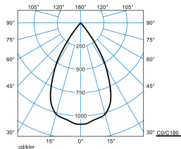
E-Line PRO 78 BV G2 RF-VFL 40-EC M39 ET 05 Blank
