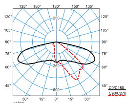
Publisca P3-AB2L-SLR3/6800-740 6G1 ET (CLO end value)
