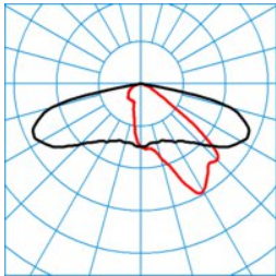
Jovie 50-AB2L-2-22-730-CLO-E
