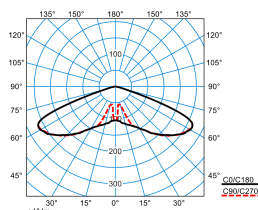
Publisca P2-RB6L-LR/1650-730 2G1S ET (CLO initial value)
