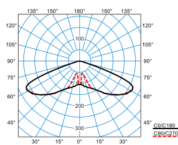
Publisca P2-RB6L-LR/1650-730 2G1S ET (CLO end value)
