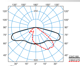
LIQ 70N-AB7L-LRA/10/12/135-727 12G1 ETDD(CLO end value) TX277745
