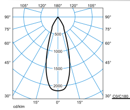
AgiraP G2 RF-FL 50-840 M43 ET 05
