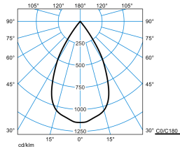
E-Line PRO 78 BV G2 RF-VFL 20-840 M35 ET 05 05
