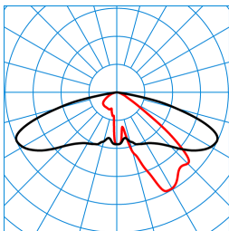
Publisca P2-AB2L-LR/4200-740 6G1S ET (CLO initial value) TX301579 ■ C0 - C180 ■ C90 - C270 DIN 5040: A30 UTE: 1,00 G DLOR: 100 % ULOR: 0 % CEN Flux Code: 35 74 97 100 100
