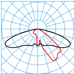
Publisca P2-AB2L-LR/4200-740 6G1S ET (CLO end value) TX300222 ■ C0 - C180 ■ C90 - C270 DIN 5040: A30 UTE: 1,00 G DLOR: 100 % ULOR: 0 % CEN Flux Code: 35 74 97 100 100
