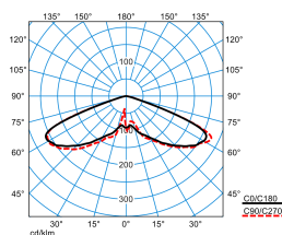
Publisca P1-RB6L/2400-740 3G1S
