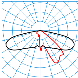
Publisca P1-AB2L/2400-740 3G1S TX047485 ■ C0 - C180 ■ C90 - C270 DIN 5040: A30 UTE: 1,00 l DLOR: 100 % ULOR: 0 % CEN Flux Code: 34 71 96 100 100
