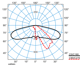
Publisca P1-AB2L/2400-740 3G1S TX047485 DIN 5040: A30 UTE: 1,00 l DLOR: 100 % ULOR: 0 % CEN Flux Code: 34 71 96 100 100
