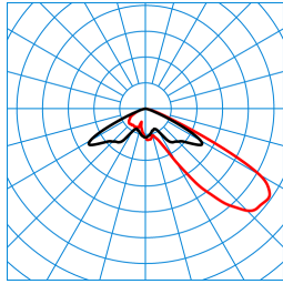
LnPlus 70-AM19L/42000-740 56G1 ETDD (CLO end value) TX377740 ■ C0 - C180 ■ C90 - C270 DIN 5040: A30 UTE: 1,00 J DLOR: 100 % ULOR: 0 % CEN Flux Code: 26 78 99 100 100
