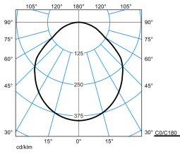
Inplana C09 OTA25 3000-830 ETDD 01 TX772695
