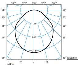
Inplana C09 OTA25 3000-830 ETDD 01 + C09 ZPF - T TX772684
