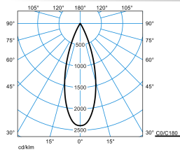
E-Line PRO 78 Lentyp L-FL 40-830 M33 ETBLE 05 05
