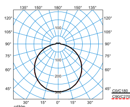
Olisq QWD3 DW 30-840 ETBLE +CAS IP54 + Olisq QWD3 ZDR 1/2 01
