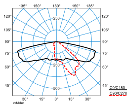
9301K AB2L-SLR2/3200-740 4G3 ET(CLO end value)
