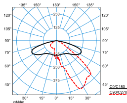
Publisca P1-AB2L-LRA/3500-730 4G1S TX047566 DIN 5040: A30 UTE: 1,00 G DLOR: 100 % ULOR: 0 % CEN Flux Code: 35 73 97 100 100
