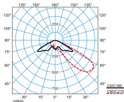
LnPlus 60-AM19L-SLR3/24000-722 18G1 ET (CLO initial value)
