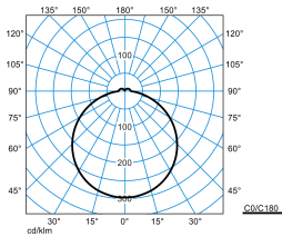
Olisq RWD3 DW 50-840 ET HFS IP54 PC + Olisq RWD3 ZDR 1/2 05
