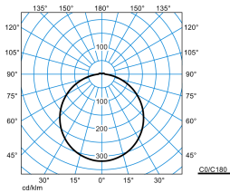
Olisq RWD3 DW 50-840 ET HFS IP54 PC + Olisq RWD3 C 01
