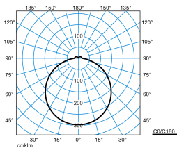
Olisq RWD3 DW 50-840 ET HFS IP54 PC + Olisq RWD3 ZDR 1/2 03
