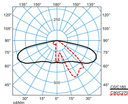
Publisca P2-AB2L-LR/1650-740 2G1S
