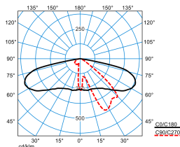
Publisca P2-AB2L-LR/1650-740 2G1S ET (CLO end value)
