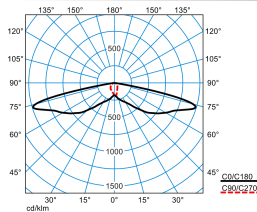
Publisca P3-SB3L-SLR3/2200-730 2G1 ET (CLO initial value)
