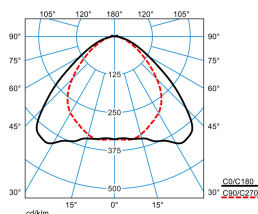
ELINE LVW55-140 ML 840 L225 4 20
