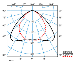
ELINE LVW55-140 ML 840 L225 2 20
