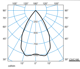
InperiaLP C05 HR19 1000-840 ET 01
