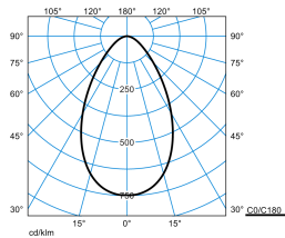
InperiaLP C05 HR19 1000-840 01 + DA-M 03
