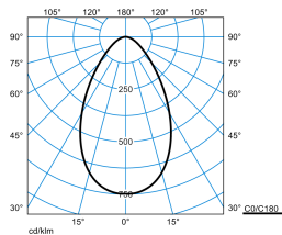
InperiaLP C05 HR19 1000-840 01 + DA-M 01
