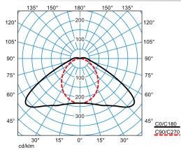
Nextrema G3 XB 40-840 ET TWP PC TX769953
