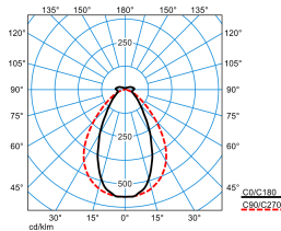
TugraHE+ 12 PN 80-830 ET PC C2
