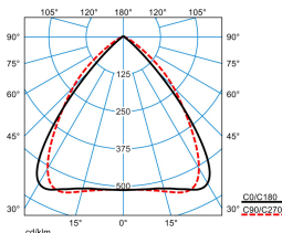
ELINE LN40-110 ML 865 L150 4 50
