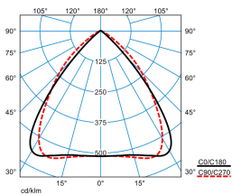
ELINE LN40-110 ML 865 L150 4 50
