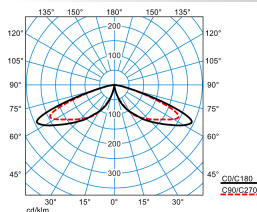
LTX LT-RB6L-LR/1200-740 2G1 ET
