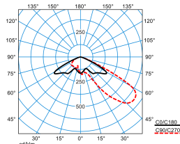
LnPlus 90-AM19L/165000-730 120G1 ETDD
