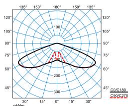
Publisca P1-RB6L-LRA/1500-730 2G1S ET (CLO initial value)
