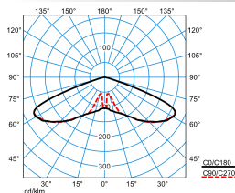
Publisca P1-RB6L-LRA/1500-730 2G1S
