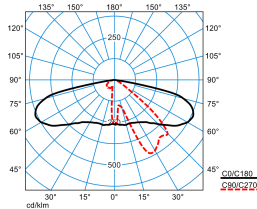
Publisca P2-AB2L-LR/1800-730 2G1S
