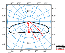
Publisca P2-AB2L-LR/1800-730 2G1S ET (CLO end value)
