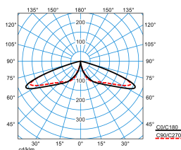
CS 19 100-RB6L-LRA/2200-740 2G1S ET (CLO end value)
