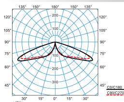
CS 19 100-RB6L-LRA/2200-740 2G1S ET (CLO initial value)
