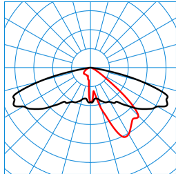
Publisca P1W-AB2L-LRA/3800-740 6G1S TX053504 ■ C0 - C180 ■ C90 - C270 DIN 5040: A30 UTE: 1,00 G DLOR: 100 % ULOR: 0 % CEN Flux Code: 34 72 97 100 100 0 0 0 0
