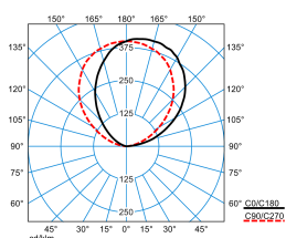
Sanesca W2 4600-8TW ETDD/ET 830 03 (DSU) (room_light)
