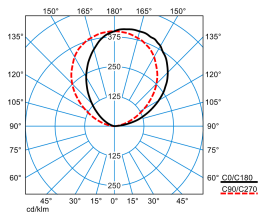
Sanesca W2 4600-8TW ETDD/ET 830 03 (DWW) (room_light)
