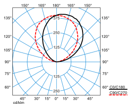
Sanesca W2 4600-8TW ETDD/ET 830 03 (DWW)
