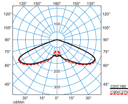
Publisca P1-RB6L-LR/3800-740 6G1S ET (CLO initial value)
