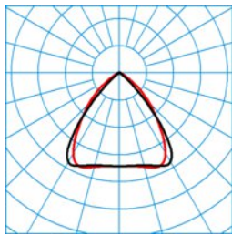
ELINE FL LN140 840 L225 1 20
