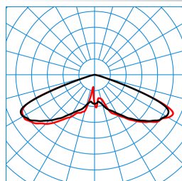
Publisca P2-RB6L-LR/2400-730 3G1S TX047860 ■ C0 - C180 ■ C90 - C270 DIN 5040: A20 UTE: 1,00 J DLOR: 100 % ULOR: 0 % CEN Flux Code: 20 57 98 100 100
