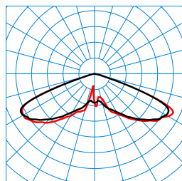
Publisca P2-RB6L-LR/2400-730 3G1S ET (CLO end value) TX301186 ■ C0 - C180 ■ C90 - C270 DIN 5040: A20 UTE: 1,00 J DLOR: 100 % ULOR: 0 % CEN Flux Code: 20 57 98 100 100
